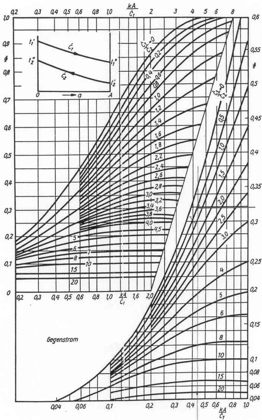
Betriebscharakteristik eines Wärmeübertragers bei Gegenstrom
