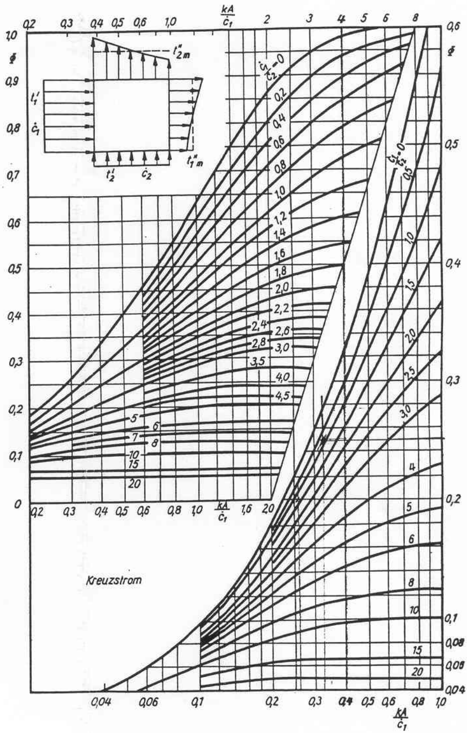
Betriebscharakteristik eines Wärmeübertragers bei Kreuzstrom
