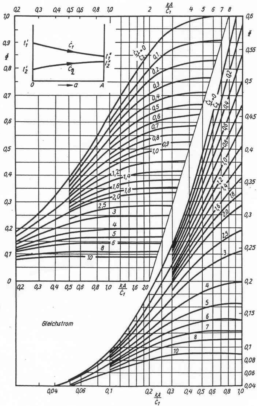
Betriebscharakteristik eines Wärmeübertragers bei Gleichstrom
